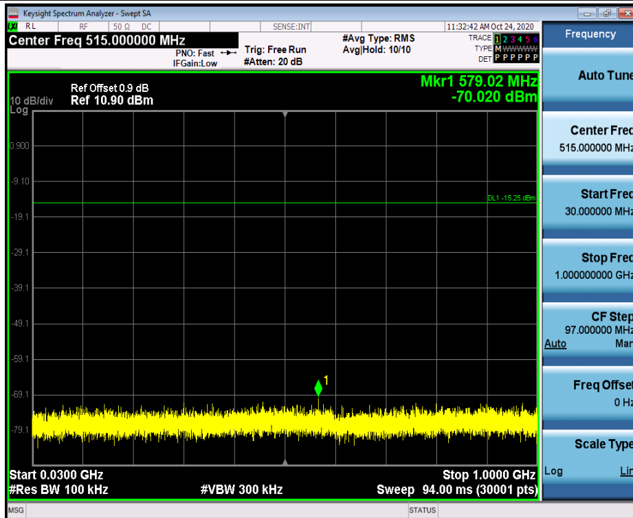
DH5_Ant1_2480_30~1000
