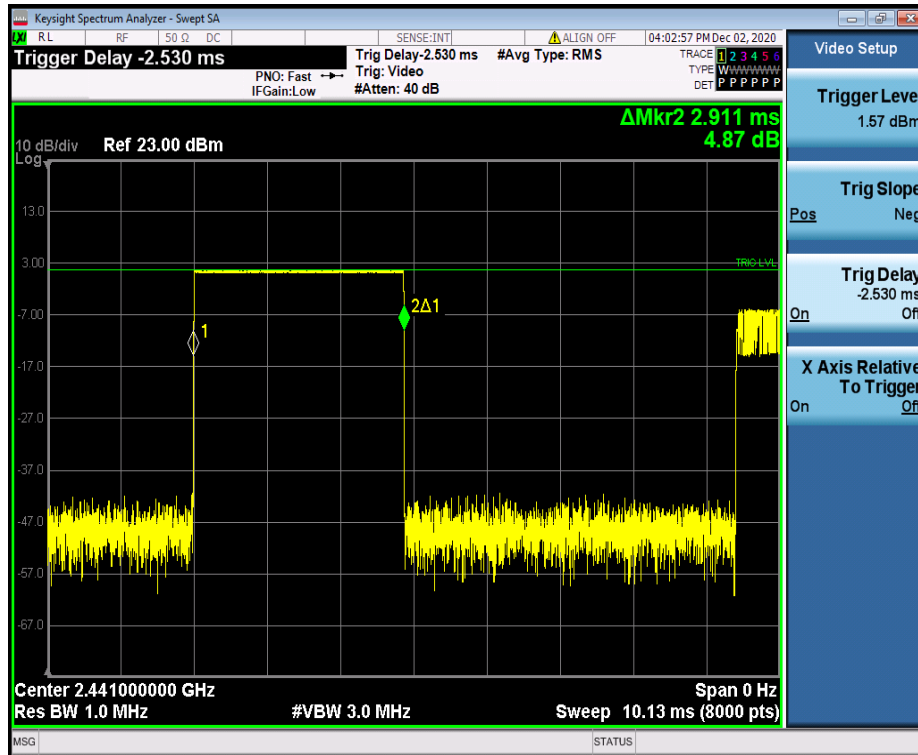
DH5_Ant1_Hop_2441
