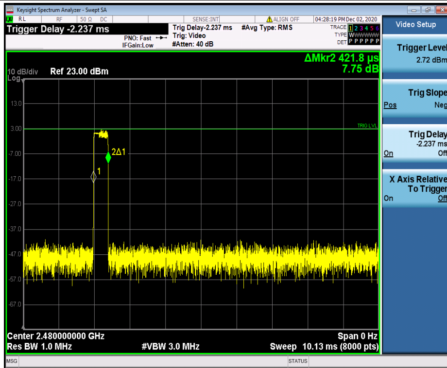
3DH1_Ant1_Hop_2480
