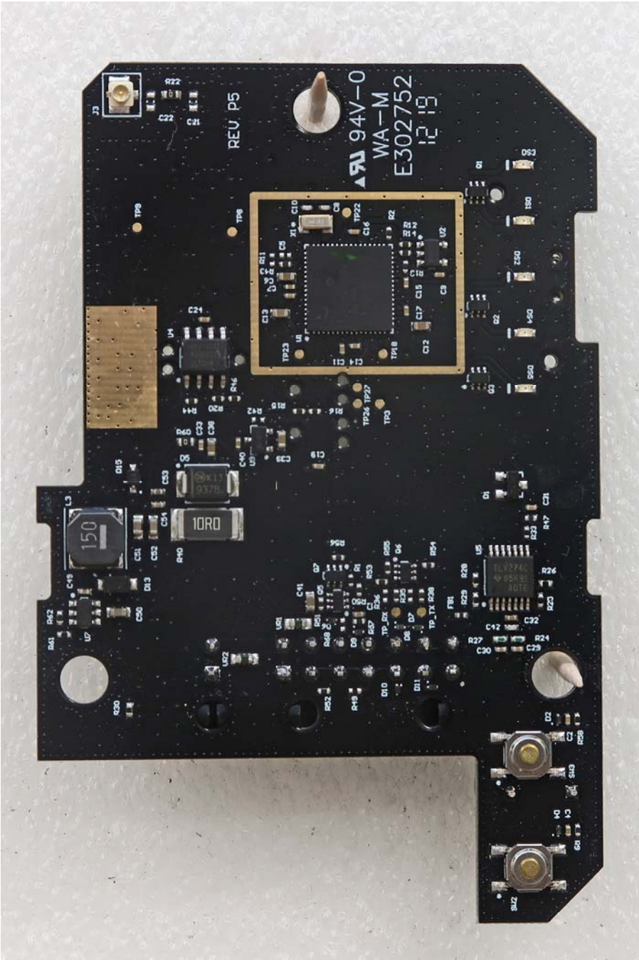
Module Front
