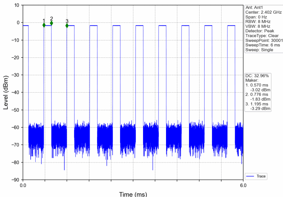
2M_LCH_2402MHz_DataRate=_Ant1_NTNV
