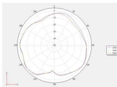
Phi 90 2D 图
