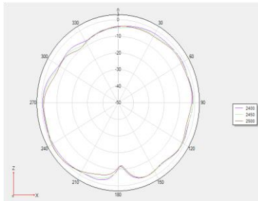
Phi 0 2D 图
