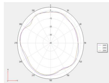
Theta 90 2D 图
