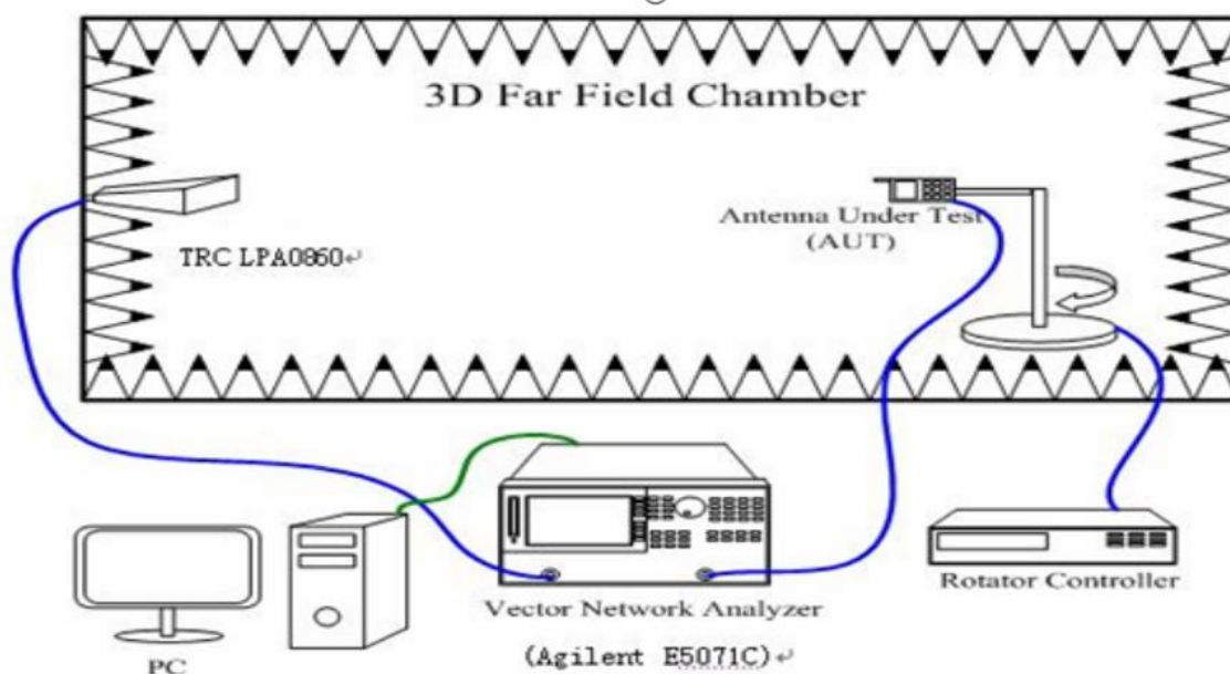
图. 1. 微波暗室内部仪器设置 r.
