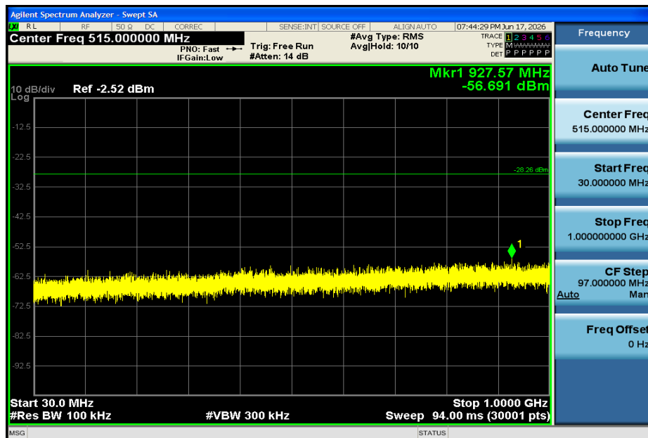
11G-Ant1-2437-30~1000-PASS
