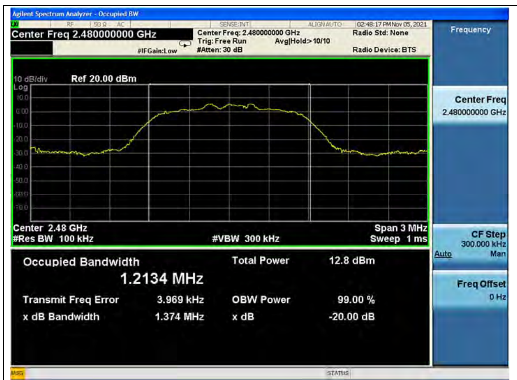
(Channel 78, \pi/4 -DQPSK)
