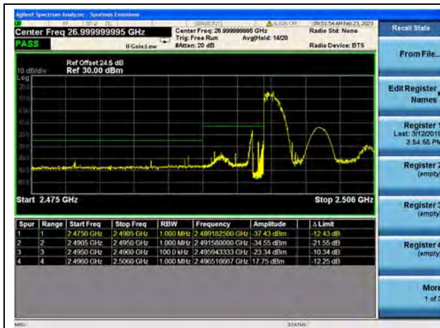
Band41 / 10MHz / Low CH / QPSK / 1 RB
