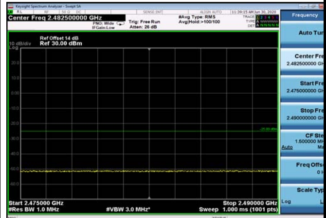
FDD07_20MHz_2560_QPSK_OneRB_low _ExtraBands_Range_2475~2490
