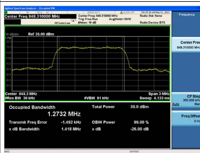
CDMA BC0 (1xRTT), CH777, 848.31MHz
