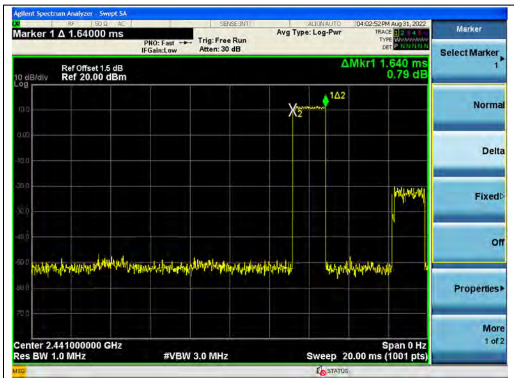
(DH3, 8-DPSK)
