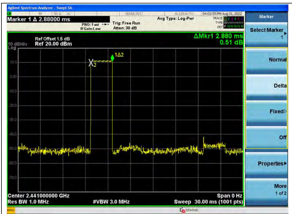
(DH5, 8-DPSK)
