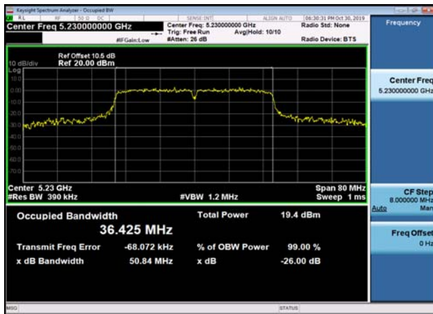
U-NII-1 26dB Bandwidth-802.11ac(40MHz),5230MHz,Ant1
