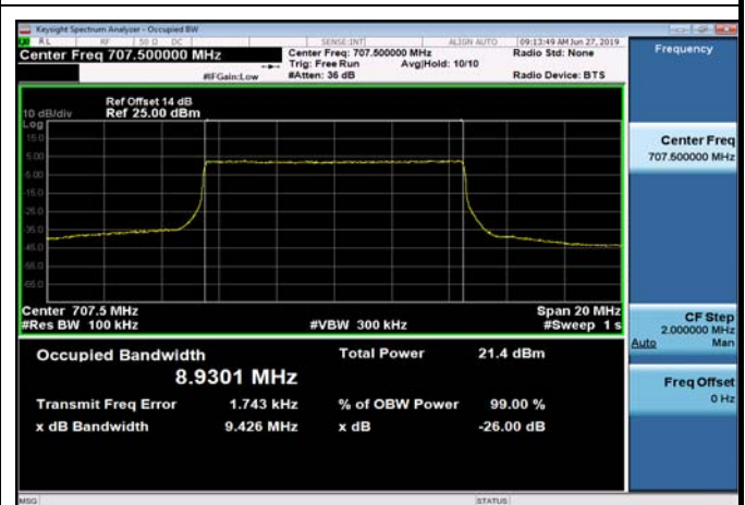
FDD12_MidRange_10MHz_707.5MHz_Q16
