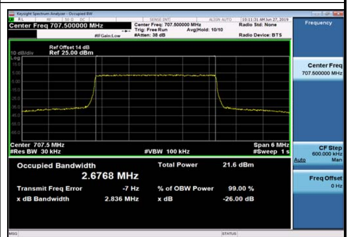
FDD12_MidRange_5_707.5_Q16
