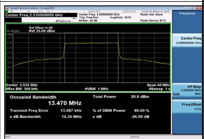
FDD07_MidRange_20_2535_Q16
