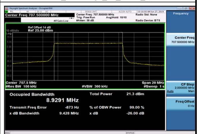
FDD12_MidRange_10_707.5_Q16
