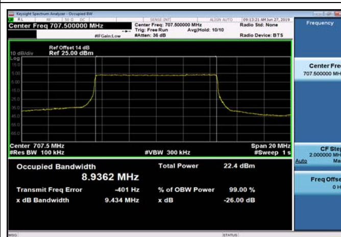
FDD12_MidRange_10MHz_707.5MHz_QPSK
