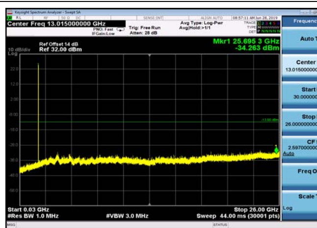
FDD25_HighRange_15MHz_30MHz~26GHz
