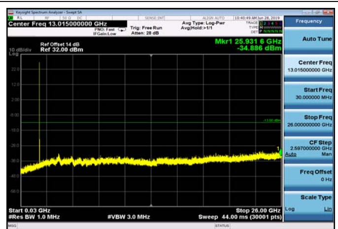
FDD25_HighRange_20MHz_30MHz~26GHz
