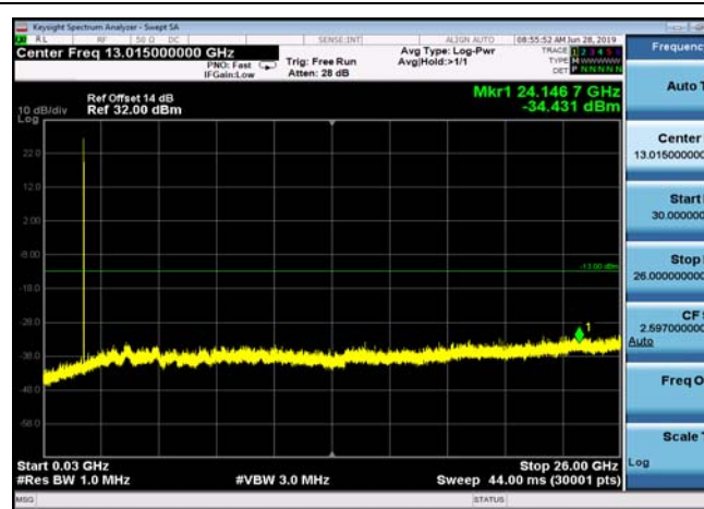
FDD25_LowRange_15MHz_30MHz~26GHz
