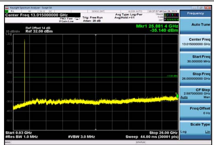
FDD25_LowRange_20MHz_30MHz~26GHz
