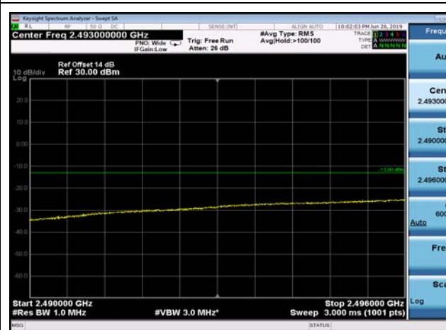
FDD07_15MHz_2507.5_Q16_fullRB_ExtraBa nds_Range_2490~2496
