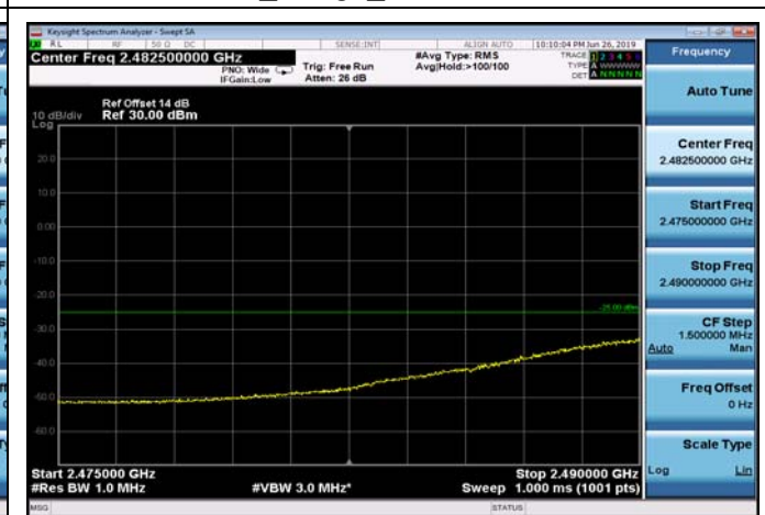
FDD07_20MHz_2510_Q16_fullIRB_ExtraBands_Range_2475~2490
