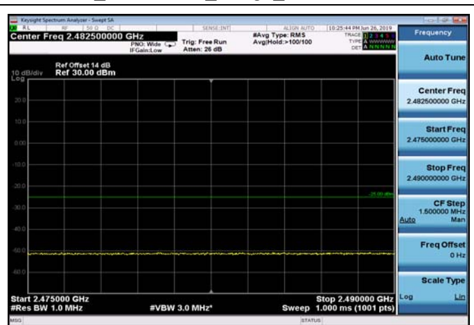
FDD07_10MHz_2565_QPSK_OneRB_low _ExtraBands_Range_2475~2490
