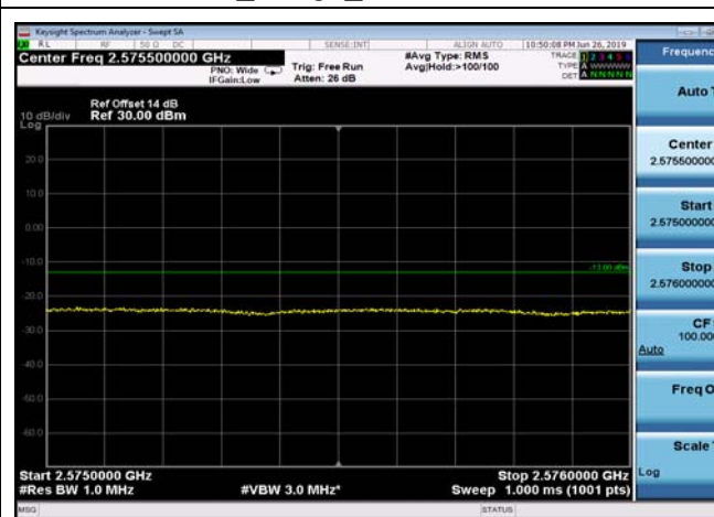
FDD07_20MHz_2560_QPSK_fullIRB_ExtraBan ds_Range_2575~2576
