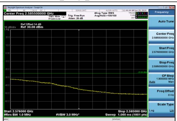
FDD07_20MHz_2560_QPSK_fullIRB_ExtraBan ds_Range_2576~2595
