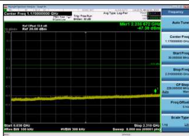
,Plot 3,30MHz~2310MHz-802.11g,2437MHz
