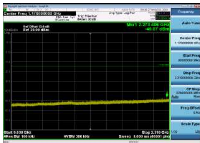
,Plot 3,30MHz~2310MHz-802.11b,2462MHz
