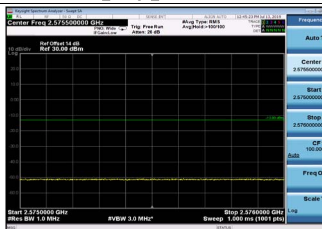
FDD07_20MHz_2510_Q16_fullRB_ExtraBand s_Range_2575~2576
