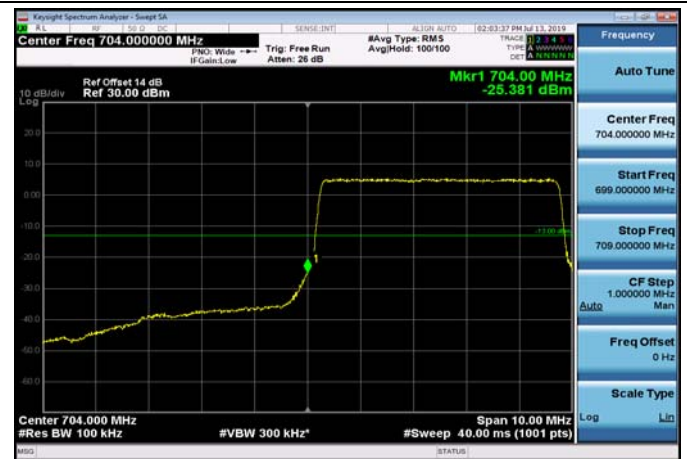
LowRange_FDD17_10MHz_709_OneRB _low_Q16
