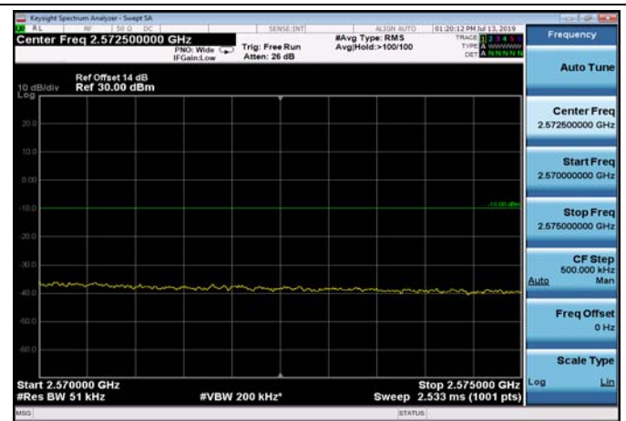
FDD07_20MHz_2560_QPSK_fullRB_ExtraBan ds_Range_2570~2575
