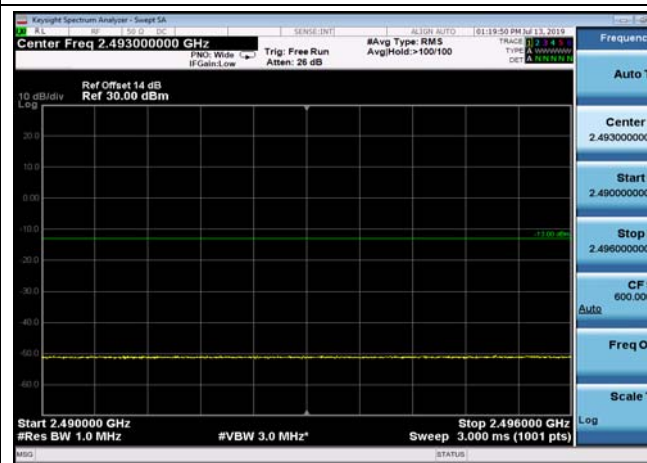
FDD07_20MHz_2560_QPSK_fullRB_ExtraBan ds_Range_2490~2496
