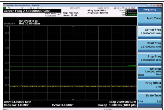
FDD07_20MHz_2510_Q16_fullRB_ExtraBand s_Range_2576~2595
