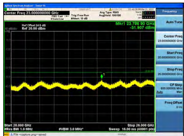
Band7-20G-26G / 5MHz / Mid CH / QPSK
