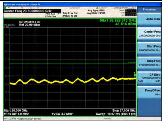
Band41-20G-27G / 5MHz / Low CH / 16QAM
