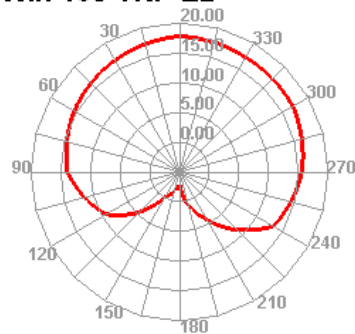
Wifi 165 TRP E2
