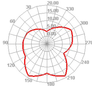
Wifi 13 TRP E2
