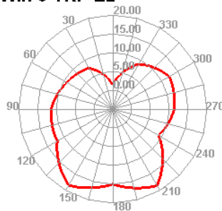
Wifi 6 TRP E2
