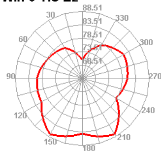
Wifi 6 TIS E2
