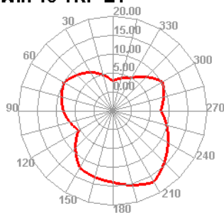
Wifi 13 TRP E1
