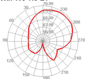
Wifi 165 TIS E1
