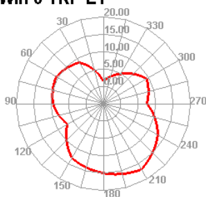
Wifi 6 TRP E1
