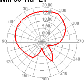
Wifi 36 TRP E1
