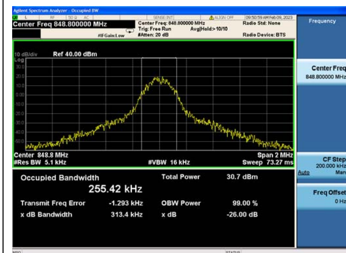
GSM850(EDGE), CH251, 848.8MHz
