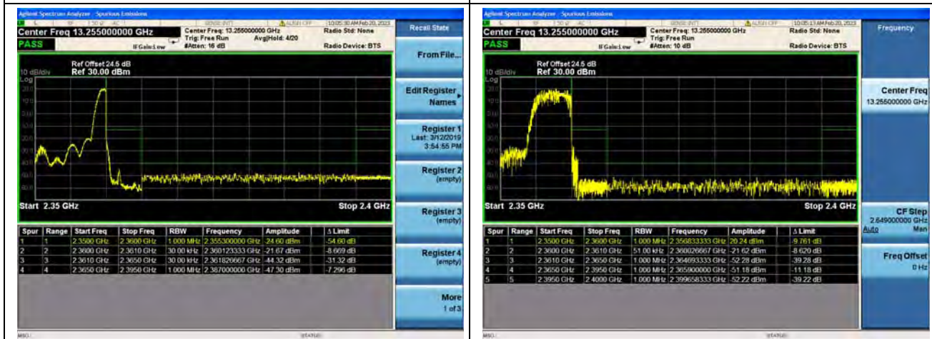
Band40 / 5MHz / High CH / QPSK / 1 RB
