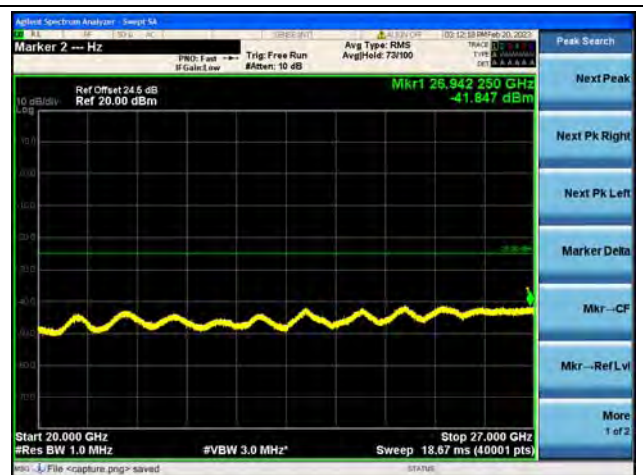
Band41(2535~2655)-20G-27G / 10MHz / High CH / QPSK
