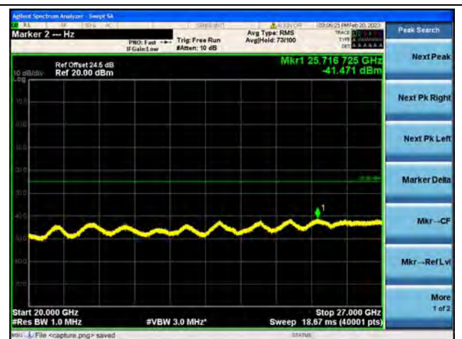
Band41(2535~2655)-20G-27G / 5MHz / Low CH / 64QAM
