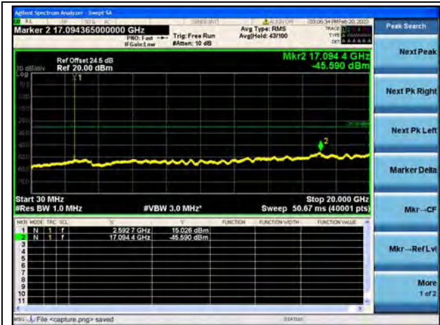
Band41(2535~2655)-30M-20G / 5MHz / Mid CH / QPSK
