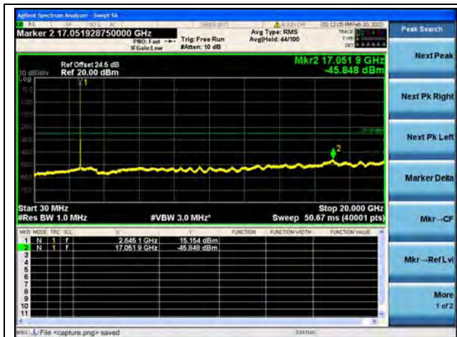
Band41(2535~2655)-30M-20G / 10MHz / High CH / QPSK
