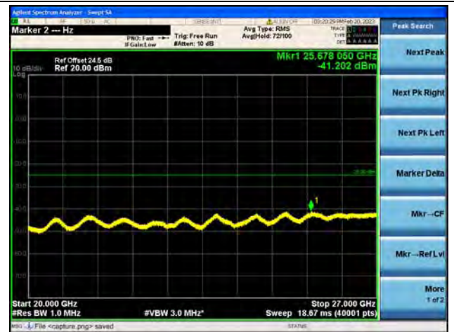
Band41(2535~2655)-20G-27G / 20MHz / High CH / 16QAM
