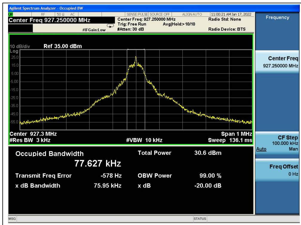
(Channel 50)
