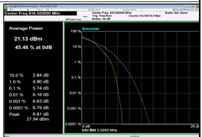
FDD26_5MHz_816.5_fullRB_Q16
