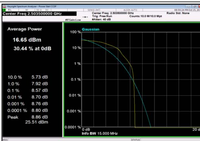
TDD41_15MHz_2503.5_OneRB_high_Q16
