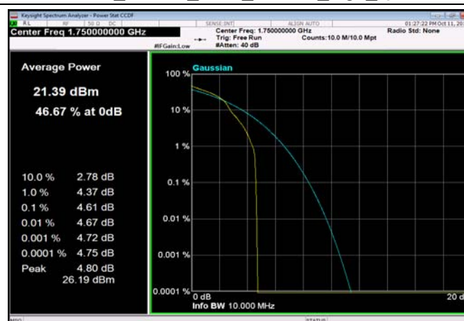
FDD04_10MHz_1750_OneRB_high_Q16
