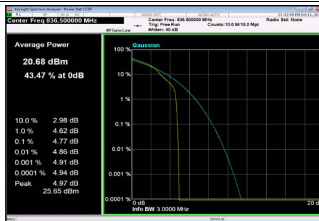
FDD05_5MHz_836.5_OneRB_high_Q16
