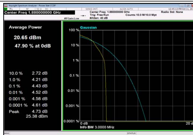
FDD02_5MHz_1880_OneRB_high_Q16
