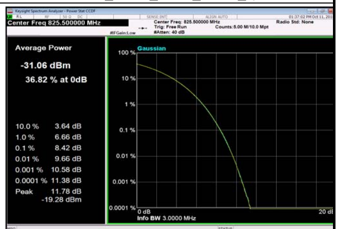
FDD05_3MHz_825.5_fullRB_Q16
