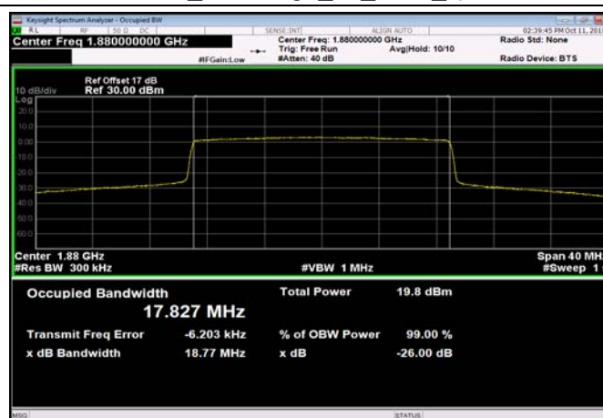
FDD02 MidRange 20 1880 Q16
