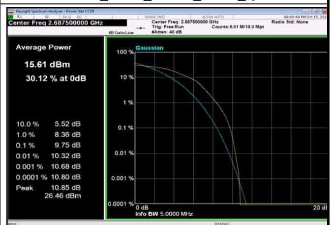
TDD41_5MHz_2687.5_fullRB_Q16
