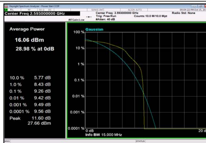
TDD41_20MHz_2593_OneRB_high_Q16
