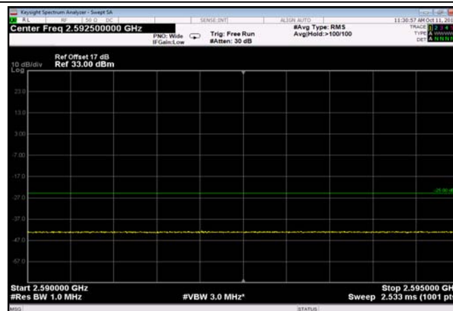
FDD07_5MHz_2567.5_Q16_OneRB_high _ExtraBands_Range_2590~2595
