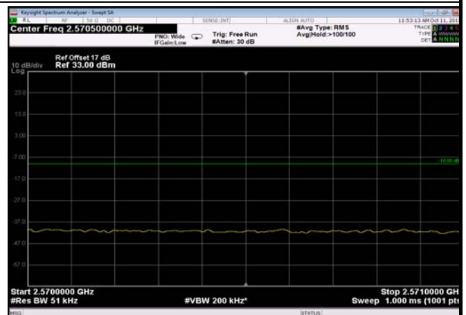
FDD07_20MHz_2560_QPSK_fullRB_ExtraBan ds_Range_2570~2571
