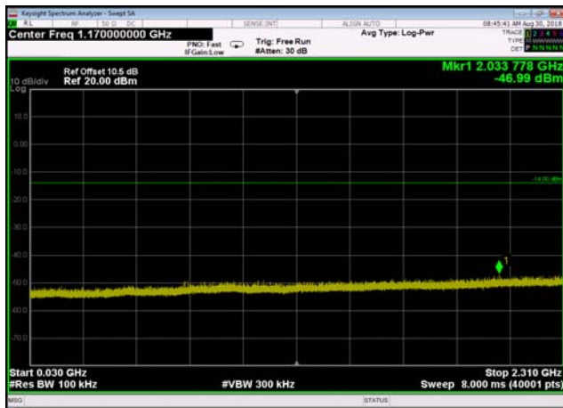
,Plot 3,30MHz~2310MHz-802.11b,2462MHz
