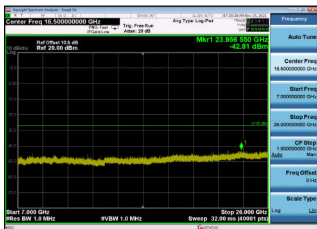
U-NII-1 ,Plot 4,7000MHz~26000MHz-802.
