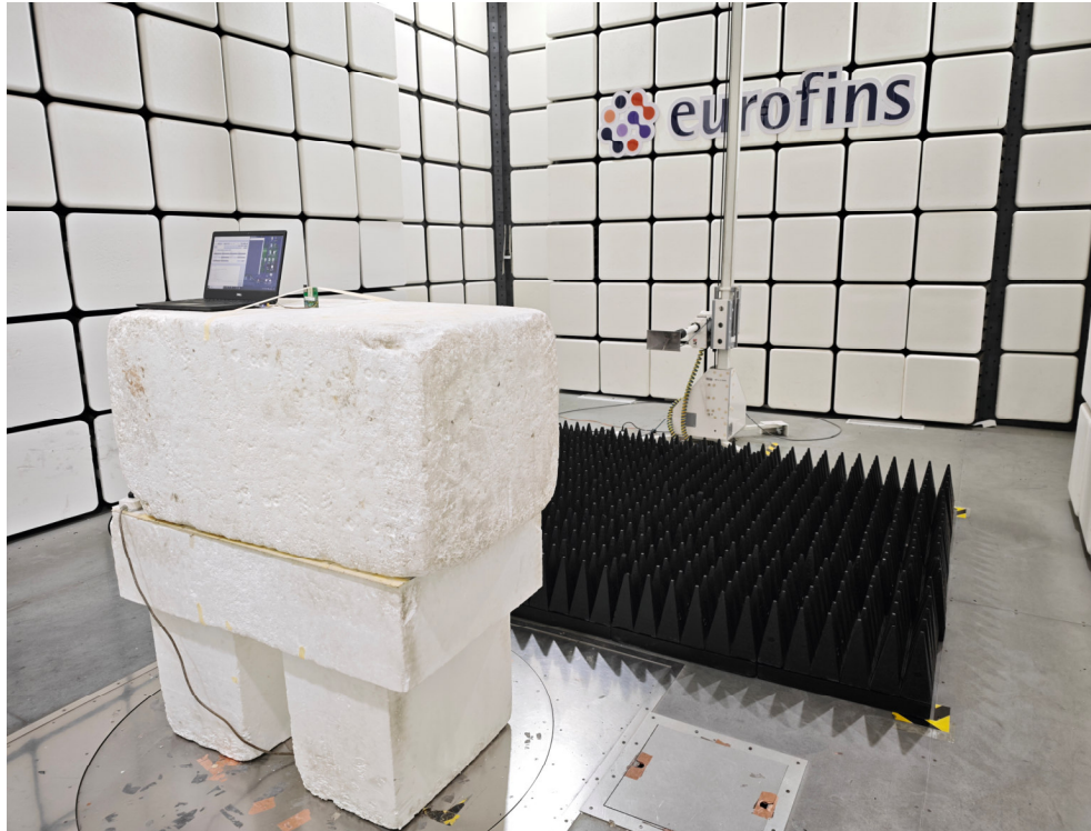
1GHz-18GHz
