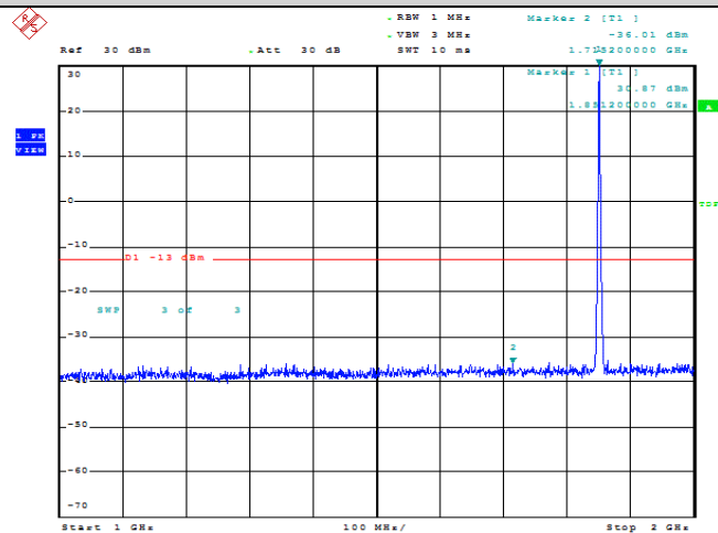
Band25-1.4MHz-QPSK-26047-1RB#0-Range2:1000~2000MHz
