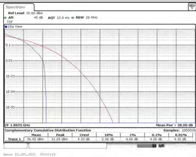
Band25-1.4MHz-QPSK-26365-1RB#0
