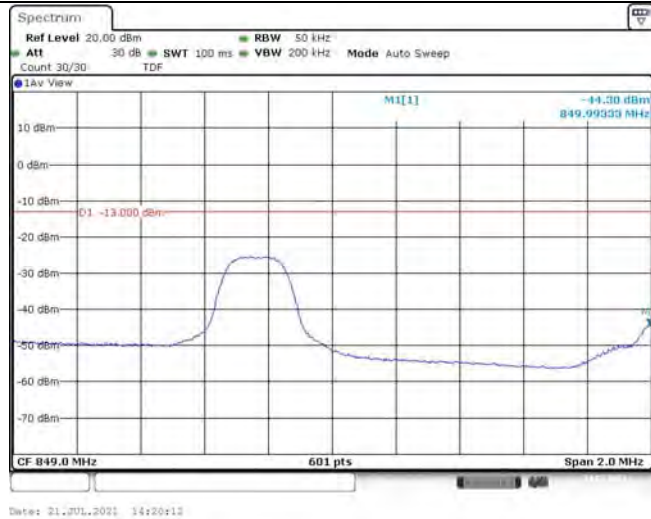
Band5-3MHz-QPSK-20635-1RB#14
