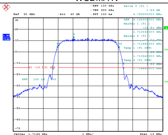
WCDMA IV
