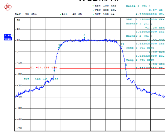
WCDMA II
