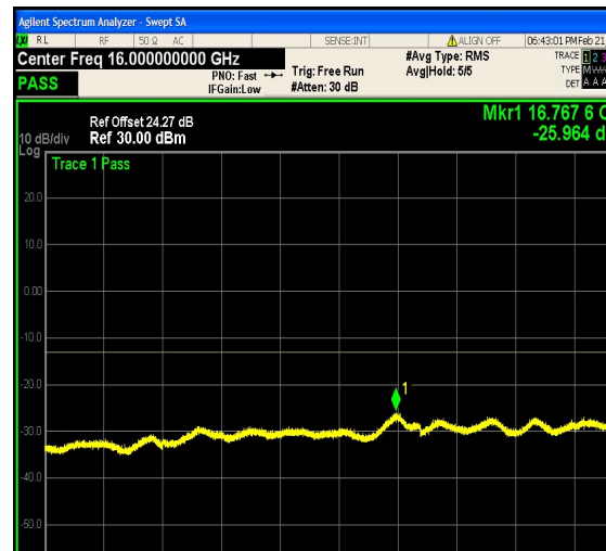
1-N66-PC3-15-10-M-25-CP-256QAM-Edge_ 1RB_Left-1@0-12000-20000-Ant1--25.96--13 -PASS
