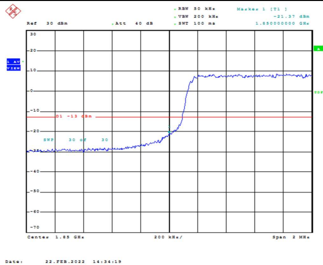
Band2-3MHz-QPSK-18615-15RB#0
