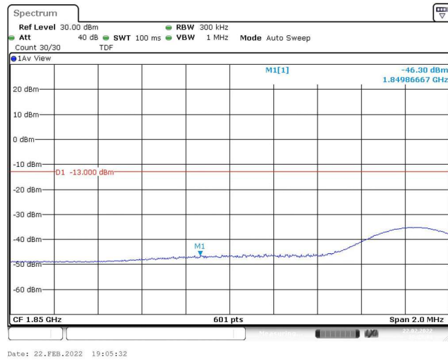
Band2-15MHz-QPSK-18675-1RB#74
