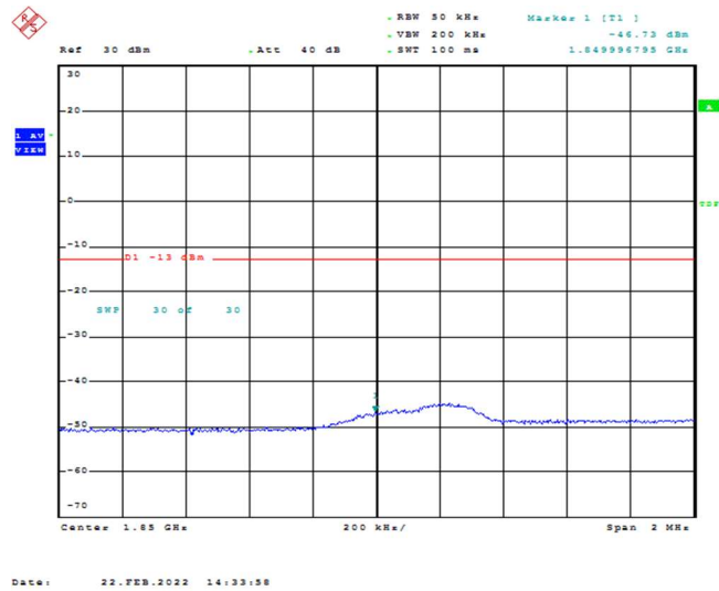
Band2-3MHz-QPSK-18615-1RB#14
