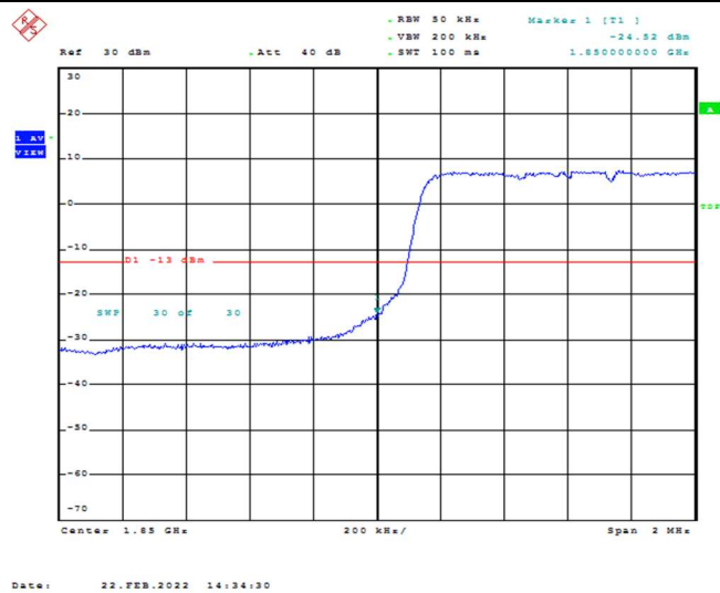
Band2-3MHz-16QAM-18615-15RB#0
