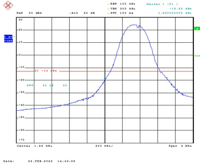
Band2-5MHz-QPSK-18625-1RB#0
