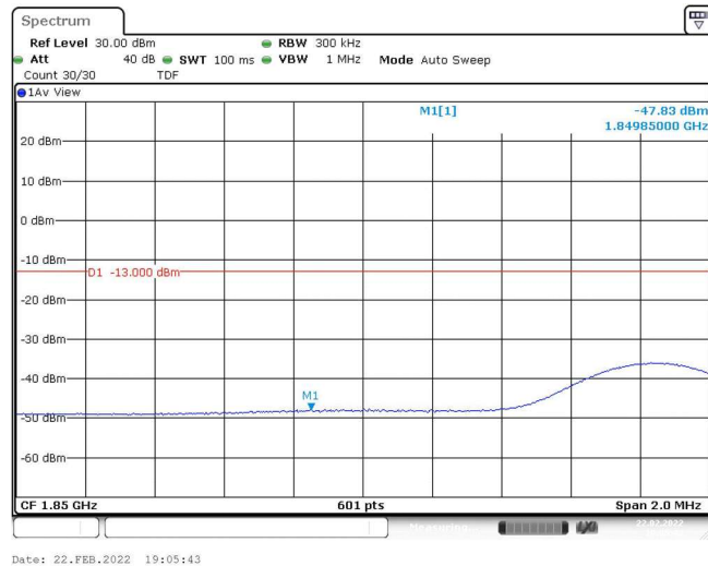
Band2-15MHz-16QAM-18675-1RB#74
