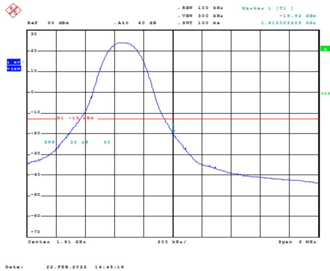
Band2-5MHz-QPSK-19175-1RB#24
