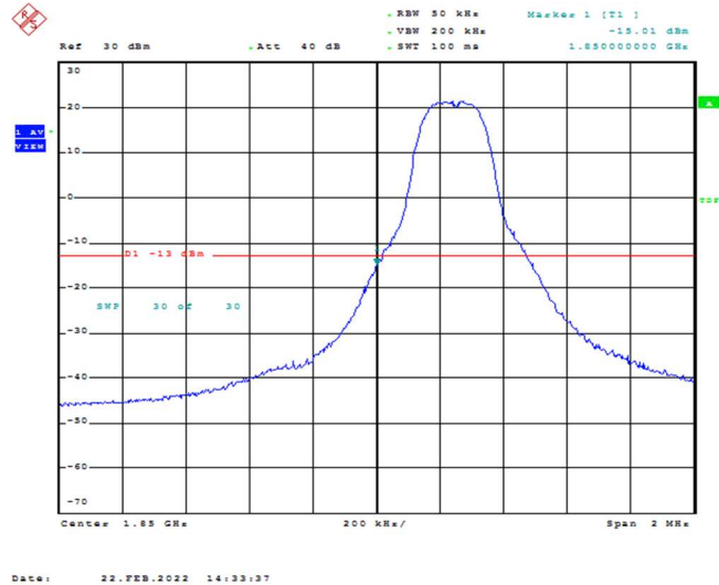
Band2-3MHz-QPSK-18615-1RB#0
