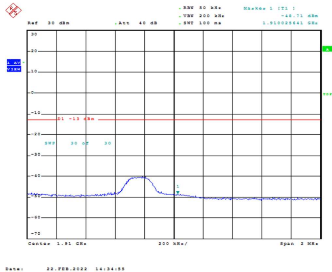
Band2-3MHz-QPSK-19185-1RB#0
