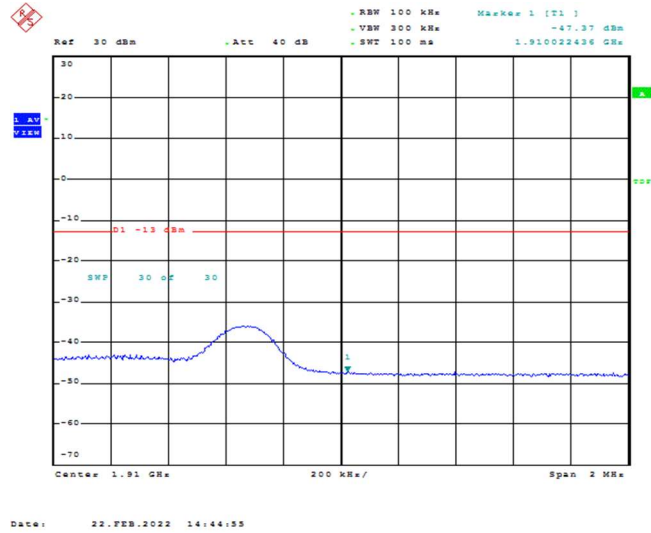
Band2-5MHz-QPSK-19175-1RB#0
