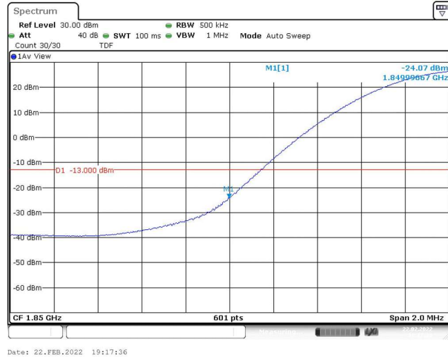
Band2-20MHz-QPSK-18700-1RB#0
