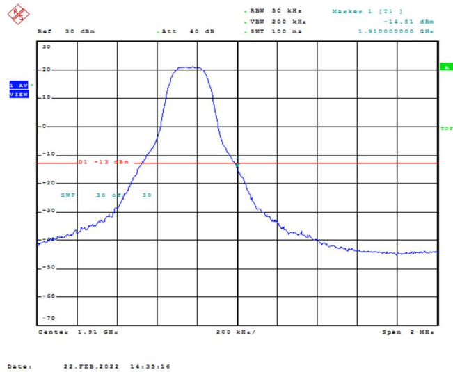
Band2-3MHz-QPSK-19185-1RB#14
