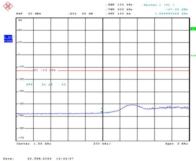
Band2-5MHz-QPSK-18625-1RB#24
