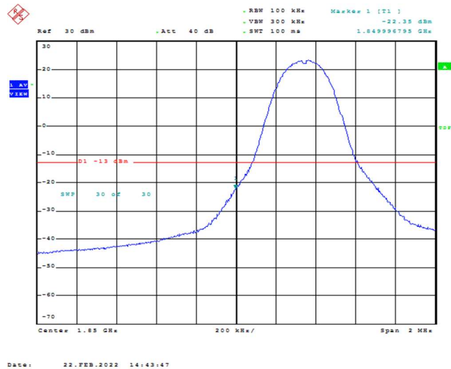
Band2-5MHz-16QAM-18625-1RB#0
