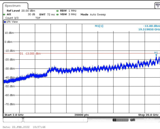
Band2-10MHz-QPSK-19150-1RB#0-Range3:2000~20000MHz
