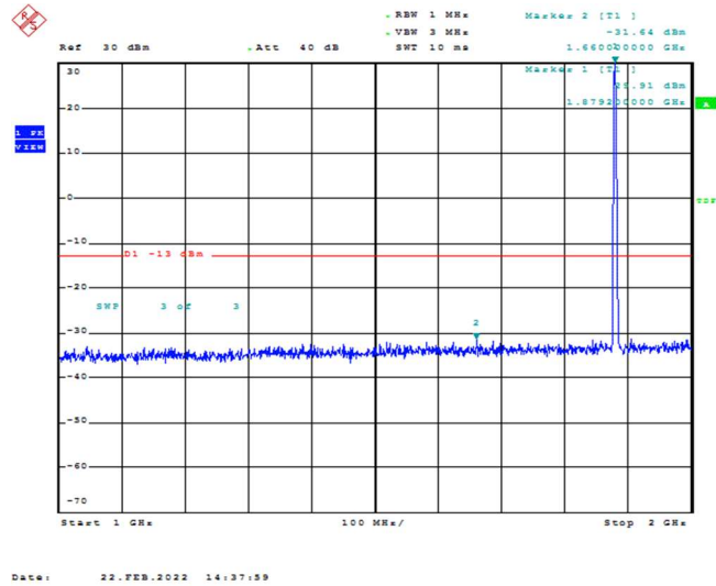
Band2-3MHz-16QAM-18900-1RB#0-Range2:1000~2000MHz
