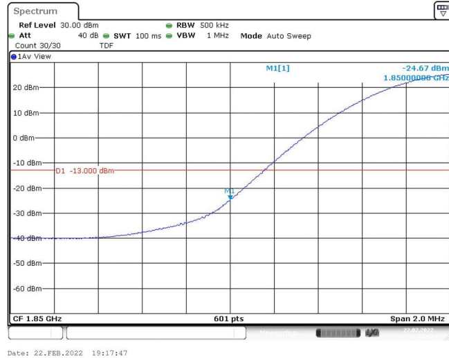
Band2-20MHz-16QAM-18700-1RB#0
