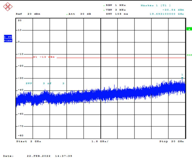
Band2-3MHz-QPSK-18900-1RB#0-Range3:2000~20000MHz
