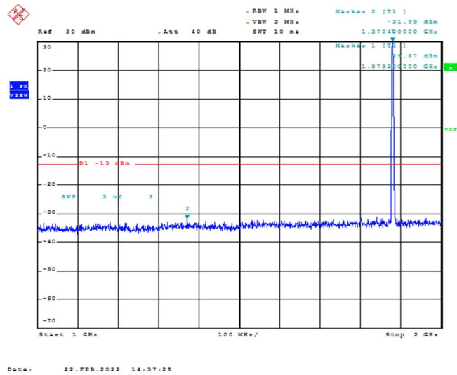
Band2-3MHz-QPSK-18900-1RB#0-Range2:1000~2000MHz
