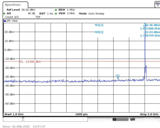
Band2-10MHz-QPSK-19150-1RB#0-Range2:1000~2000MHz
