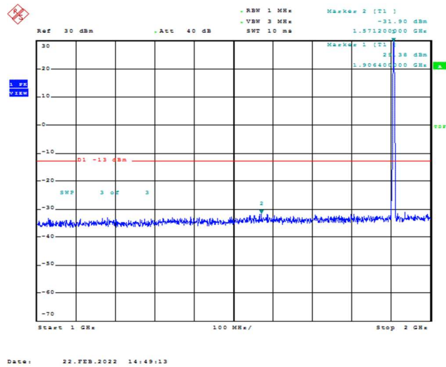
Band2-5MHz-16QAM-19175-1RB#0-Range2:1000~2000MHz
