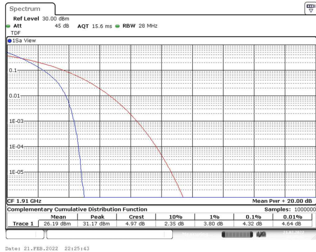
Band25-10MHz-QPSK-26640-50RB#0
