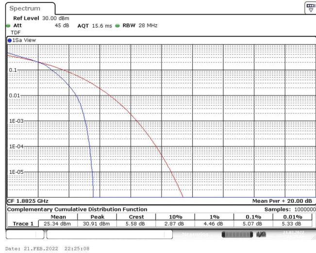
Band25-10MHz-16QAM-26365-50RB#0
