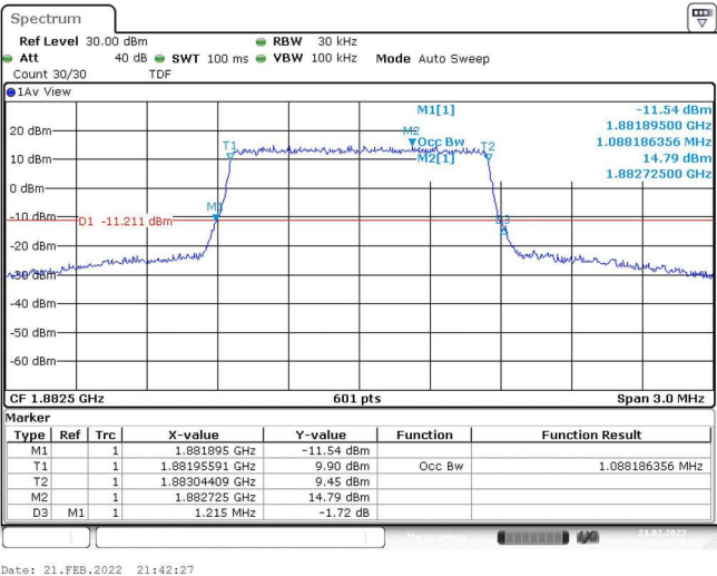
Band25-1.4MHz-QPSK-26365-6RB#0-1.088
