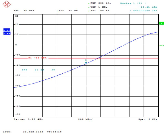
Band25-20MHz-QPSK-26140-1RB#0
