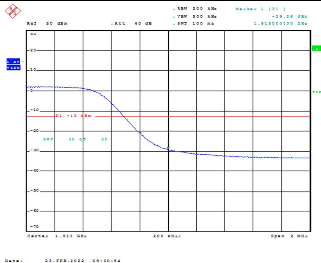
Band25-10MHz-QPSK-26640-50RB#0
