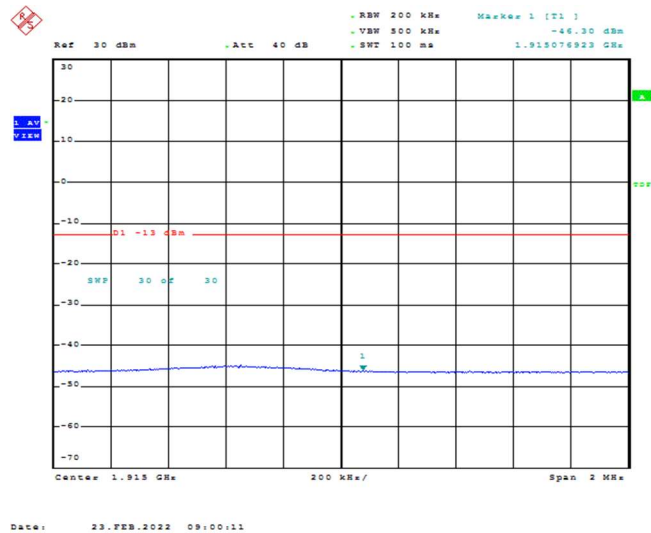
Band25-10MHz-QPSK-26640-1RB#0
