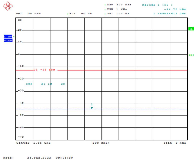
Band25-20MHz-QPSK-26140-1RB#99
