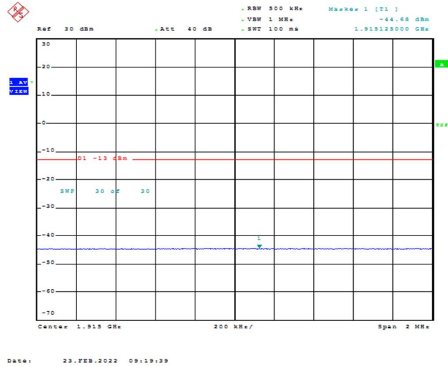
Band25-20MHz-QPSK-26590-1RB#0
