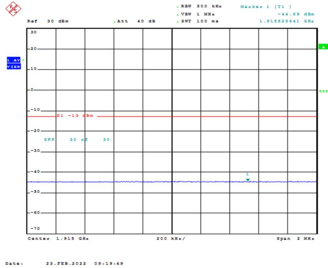
Band25-20MHz-16QAM-26590-1RB#0
