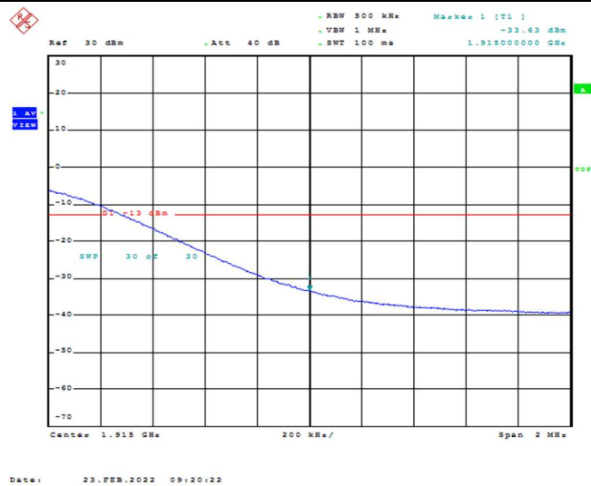
Band25-20MHz-QPSK-26590-100RB#0
