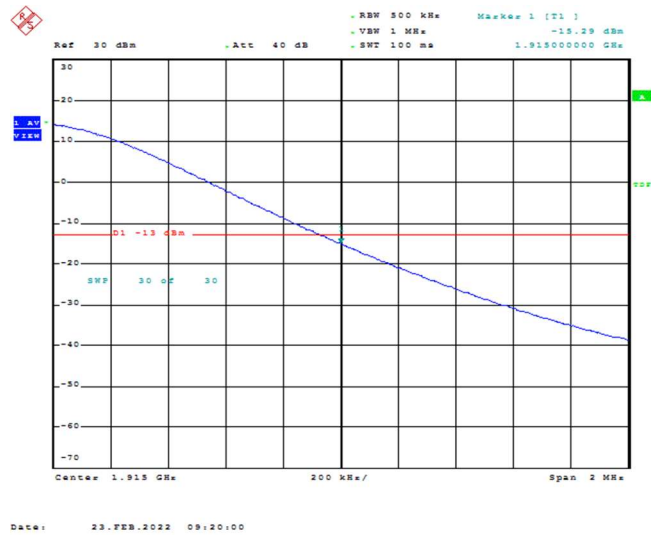
Band25-20MHz-QPSK-26590-1RB#99
