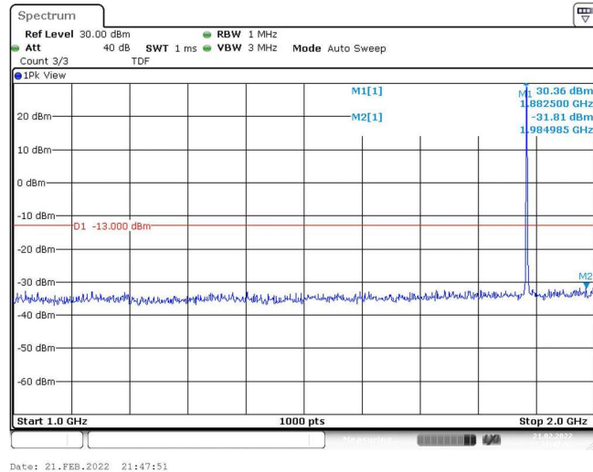
Band25-1.4MHz-QPSK-26365-1RB#0-Range2:1000~2000MHz
