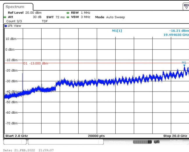
Band25-3MHz-QPSK-26365-1RB#0-Range3:2000~20000MHz
