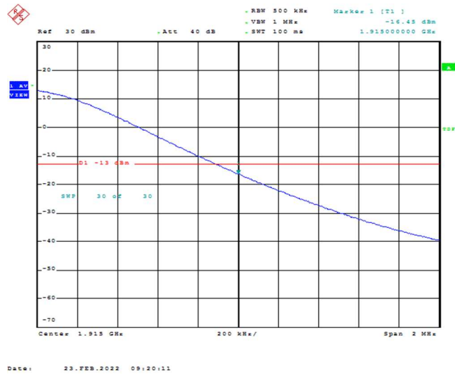
Band25-20MHz-16QAM-26590-1RB#99
