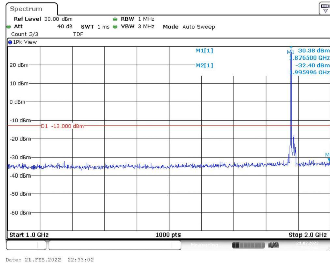
Band25-15MHz-QPSK-26365-1RB#0-Range2:1000~2000MHz
