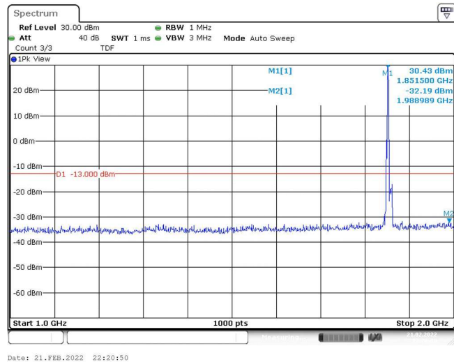
Band25-10MHz-QPSK-26090-1RB#0-Range2:1000~2000MHz
