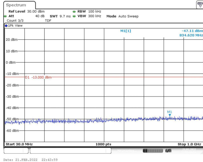
Band25-20MHz-QPSK-26365-1RB#0-Range1:30~1000MHz
