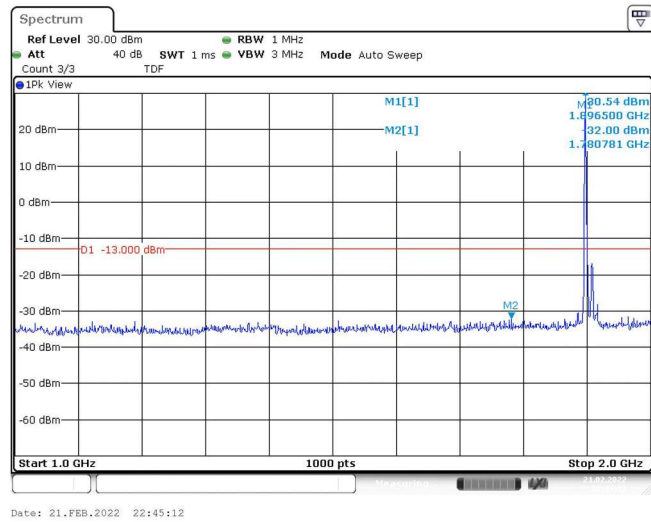
Band25-20MHz-QPSK-26590-1RB#0-Range2:1000~2000MHz
