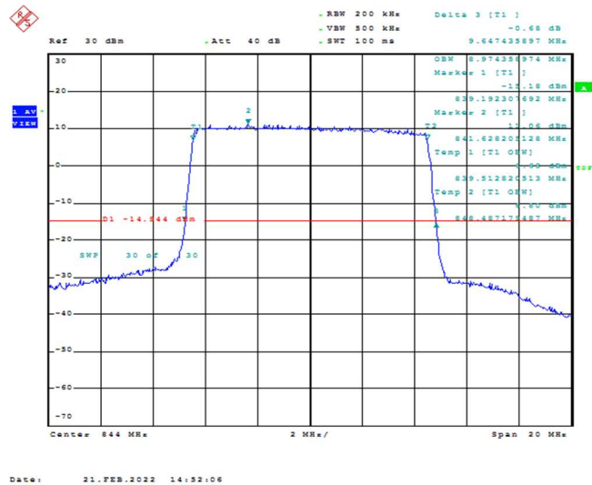
Band26-10MHz-QPSK-26990-50RB#0-8.974
