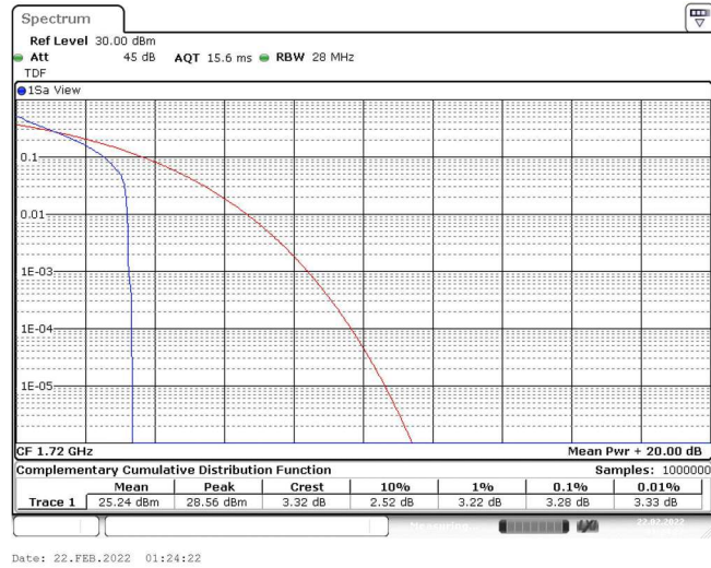
Band4-20MHz-QPSK-20050-1RB#0
