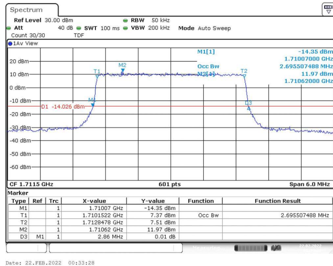
Band4-3MHz-QPSK-19965-15RB#0-2.696
