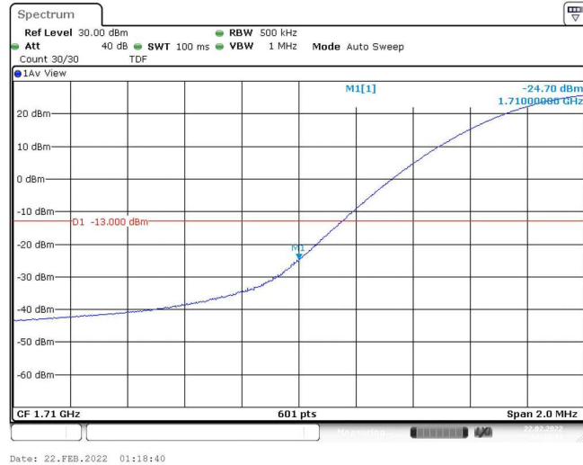
Band4-20MHz-QPSK-20050-1RB#0
