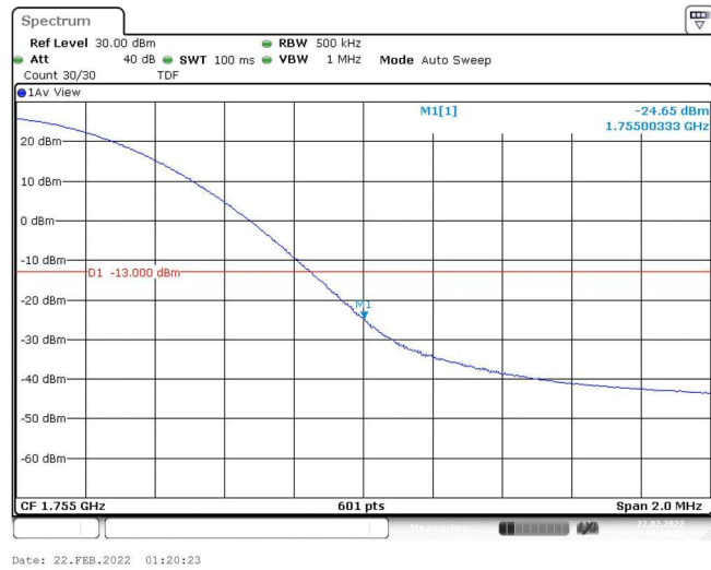
Band4-20MHz-QPSK-20300-1RB#99
