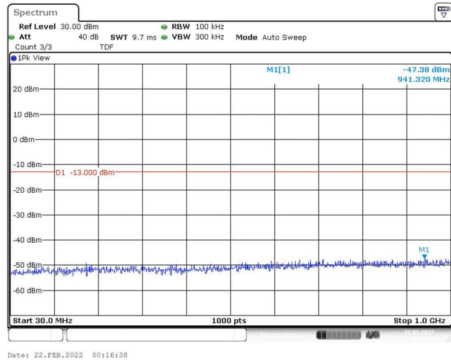
Band4-1.4MHz-QPSK-20393-1RB#0-Range1:30~1000MHz
