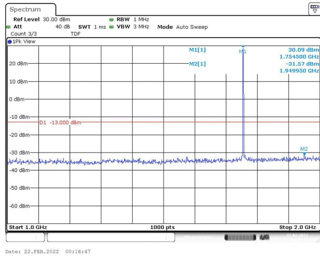
Band4-1.4MHz-QPSK-20393-1RB#0-Range2:1000~2000MHz
