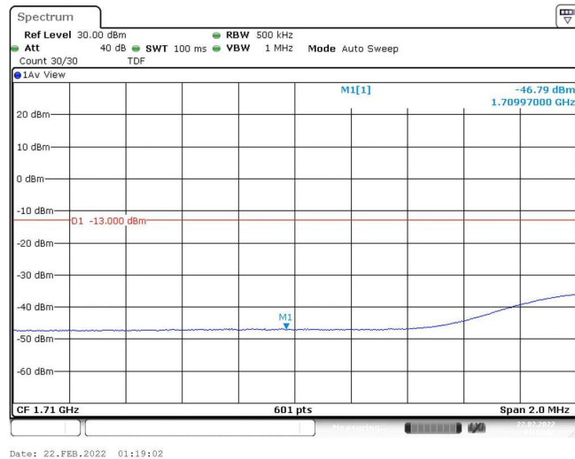
Band4-20MHz-QPSK-20050-1RB#99
