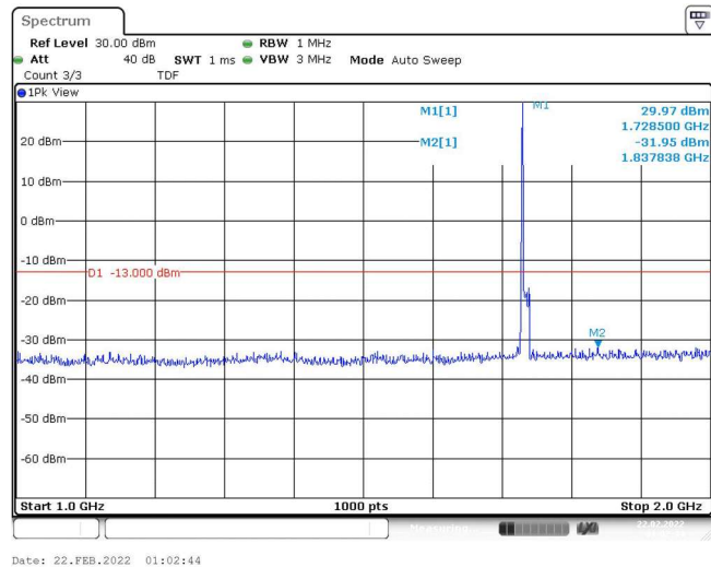
Band4-10MHz-QPSK-20175-1RB#0-Range2:1000~2000MHz
