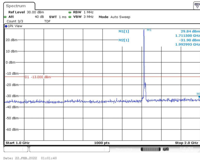
Band4-10MHz-QPSK-20000-1RB#0-Range2:1000~2000MHz
