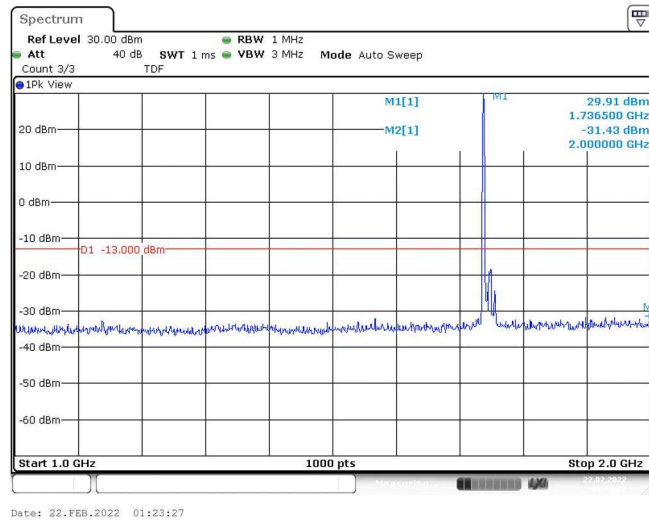
Band4-20MHz-QPSK-20300-1RB#0-Range2:1000~2000MHz
