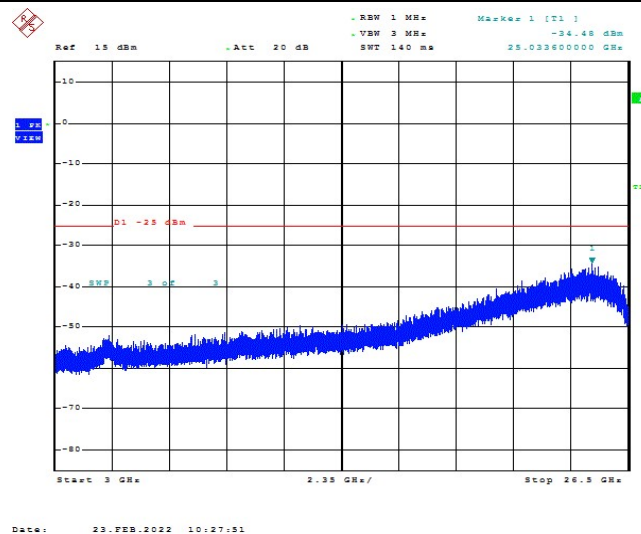
Band41-5MHz-QPSK-39675-1RB#0-Range1:3000~26500MHz
