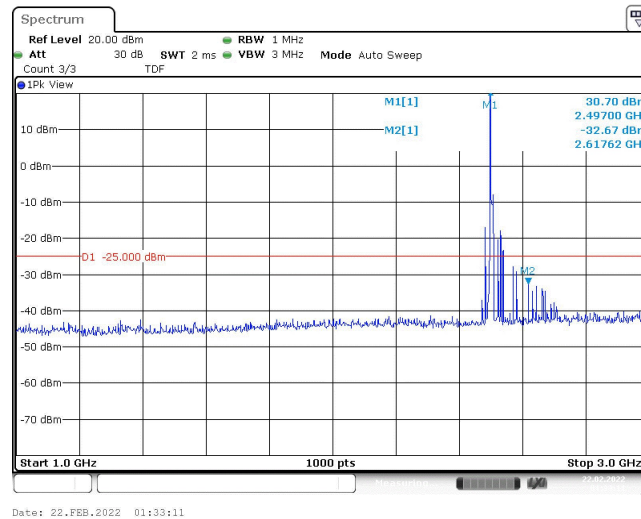
Band41-5MHz-QPSK-39675-1RB#0-Range2:1000~3000MHz
