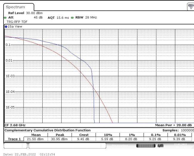
Band41-20MHz-16QAM-41490-1RB#0
